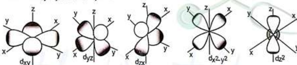
চিত্র: d-অরবিটালসমূহ
